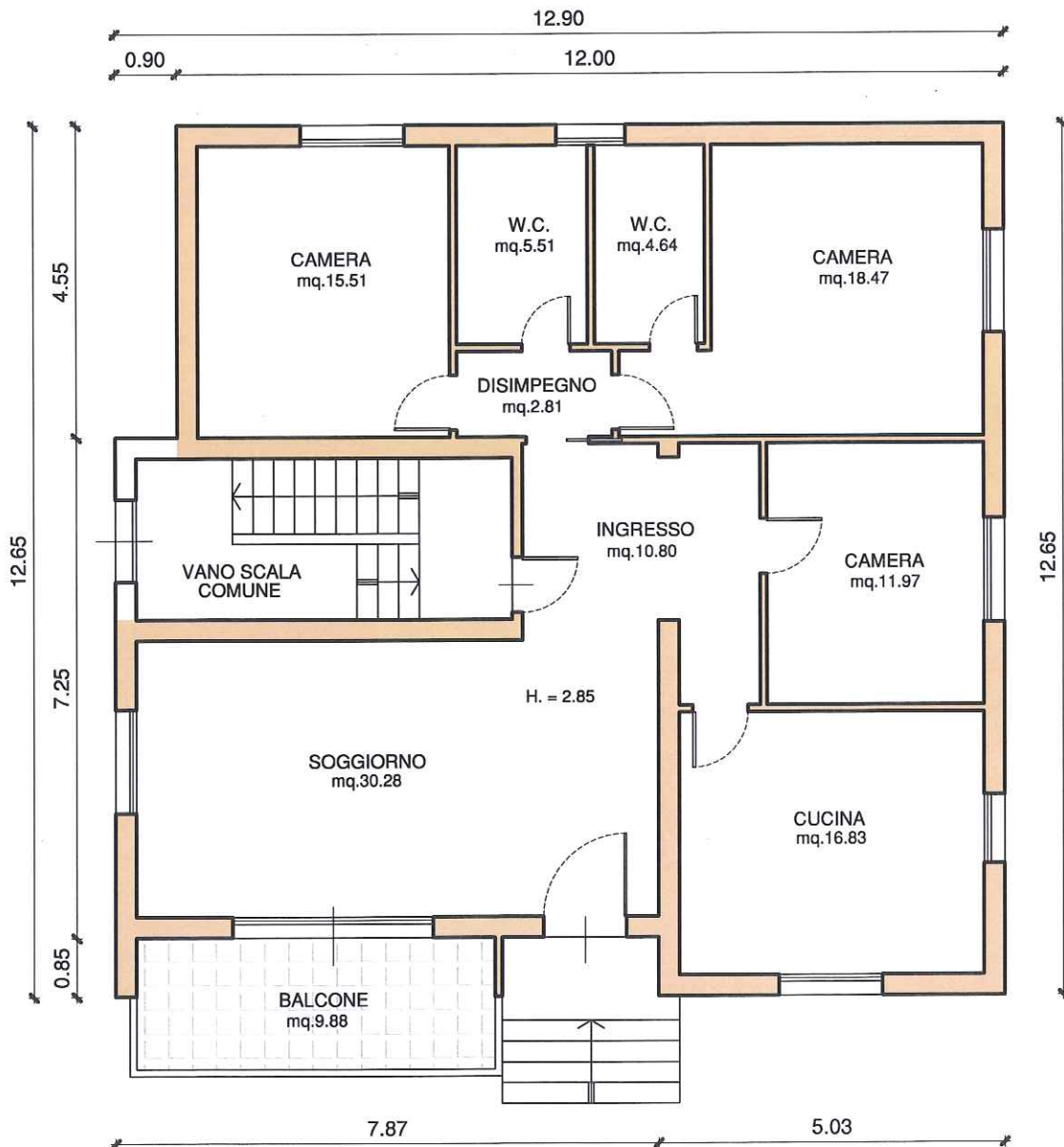
PIANTA PIANO RIALZATO - 1:100
